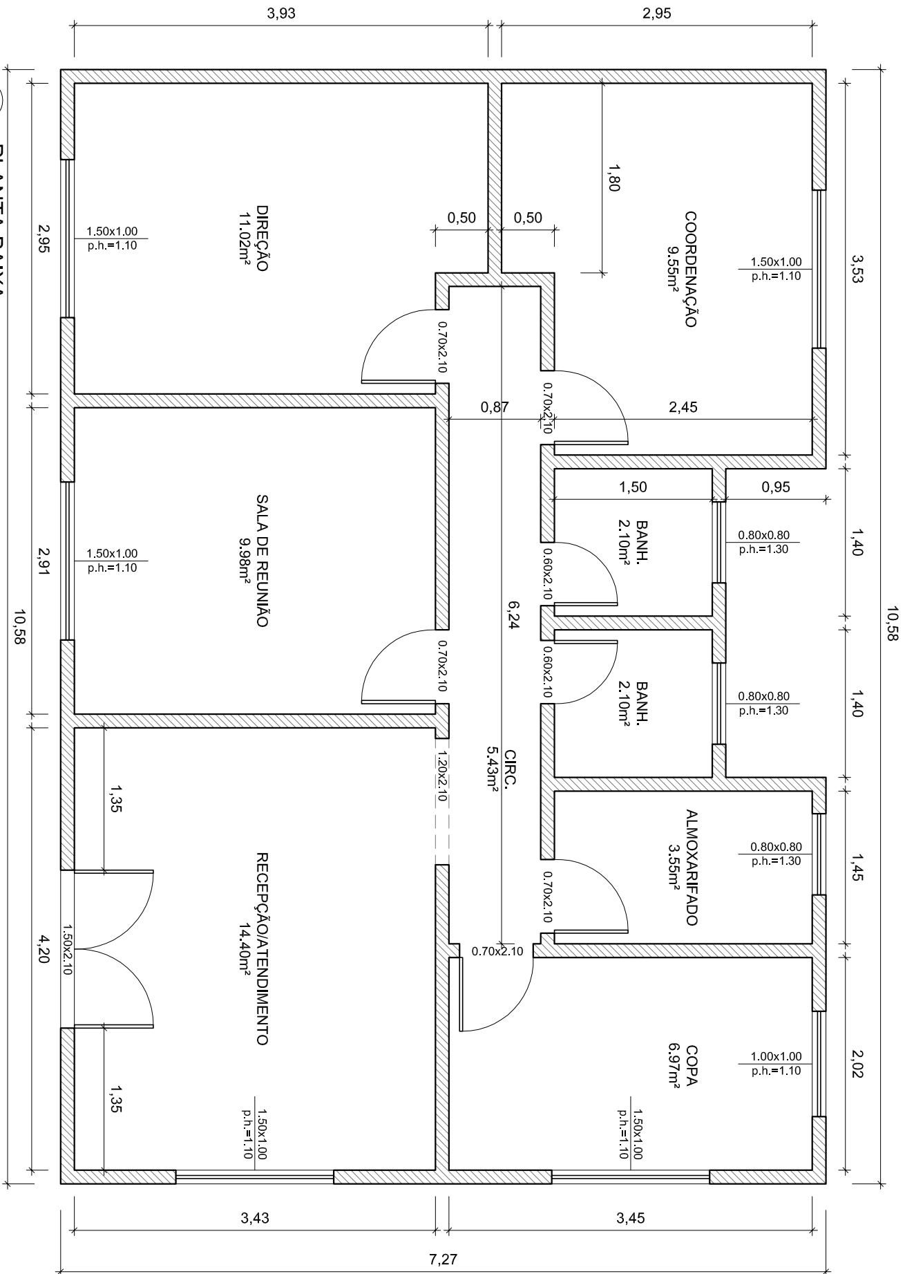
01 PLANTA BAIXA ESC:1/50
